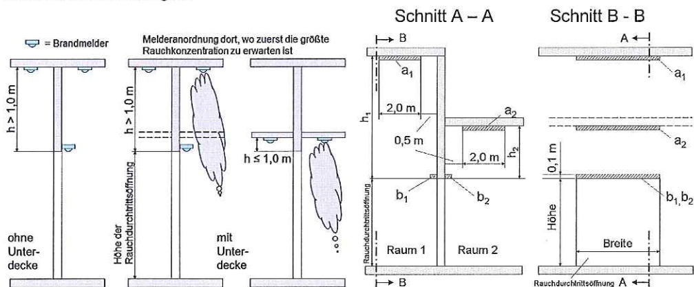
Bild 1: Maßgebende Höhe der Deckenunterfläche Bild 2: Installationsbereiche
